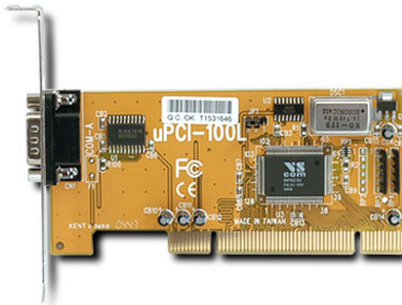
Abbildung 1: VScom 100L UPCI
